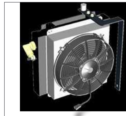
Motoventilateur avec fonction de dépoussiérage automatique. 2 seuils de détection configurables pour gérer l'activation du refroidisseur et l'arrêt du rotor, avec sonde réglable
